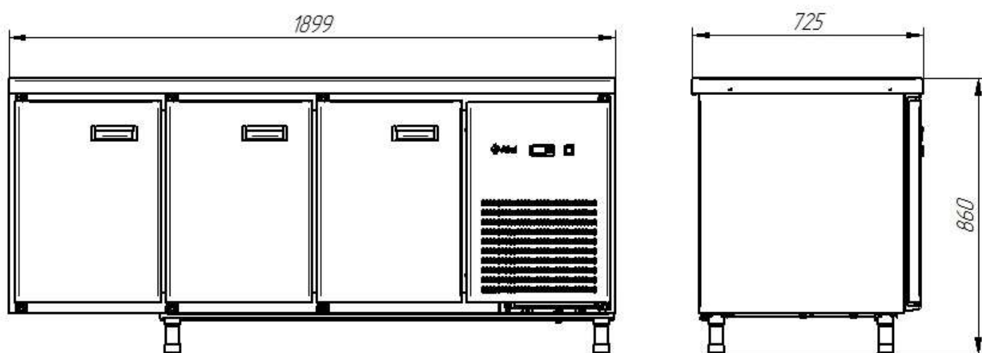
Рис.7. Габаритные размеры CXС-70-02-СО столешница без борта (дверь, дверь, дверь)*
