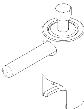
Рис. 10. Съемник для крыльчатки
