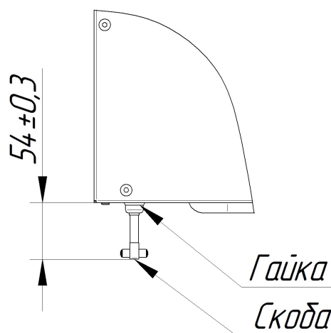
Рис. 8. Регулировка замкового устройства (для КЭП-6П-01 и КЭП-10П-01)
