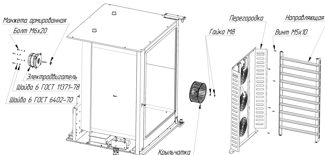
Рис. 9. Замена манжет (дверь, часть облицовки условно не показана)
