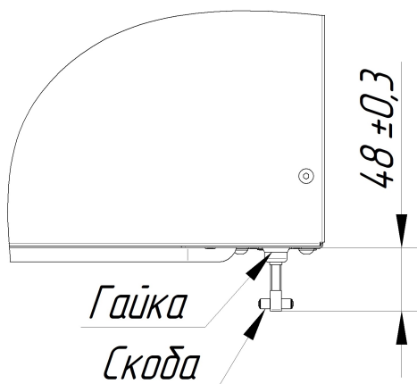
Рис. 7. Регулировка замкового устройства (для КЭП-4ПМ-01)
