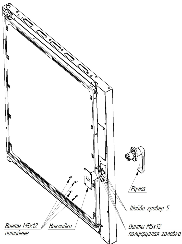
Рис. 6. Замена ручки
